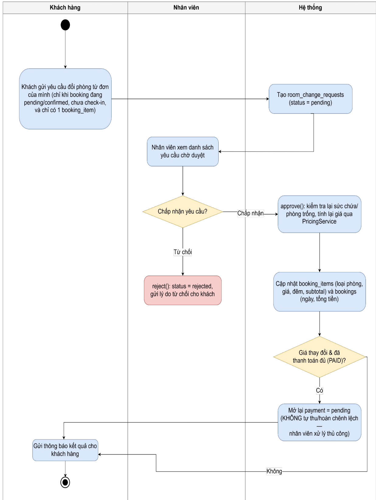
Hình 3.7.9: Sơ đồ hoạt động chức năng yêu cầu đổi phòng
