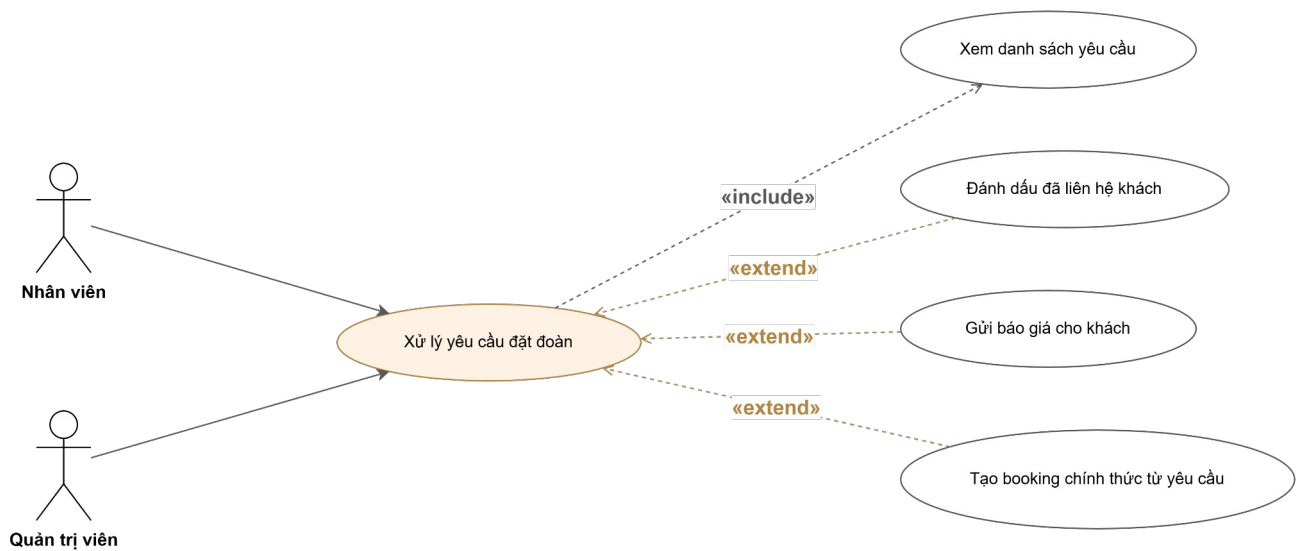
Hình 3.4.2.18: Sơ đồ Use case — Xử lý đặt đoàn / nhóm
