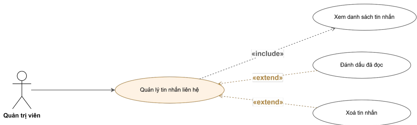
Hình 3.4.2.31: Sơ đồ Use case — Quản lý liên hệ
