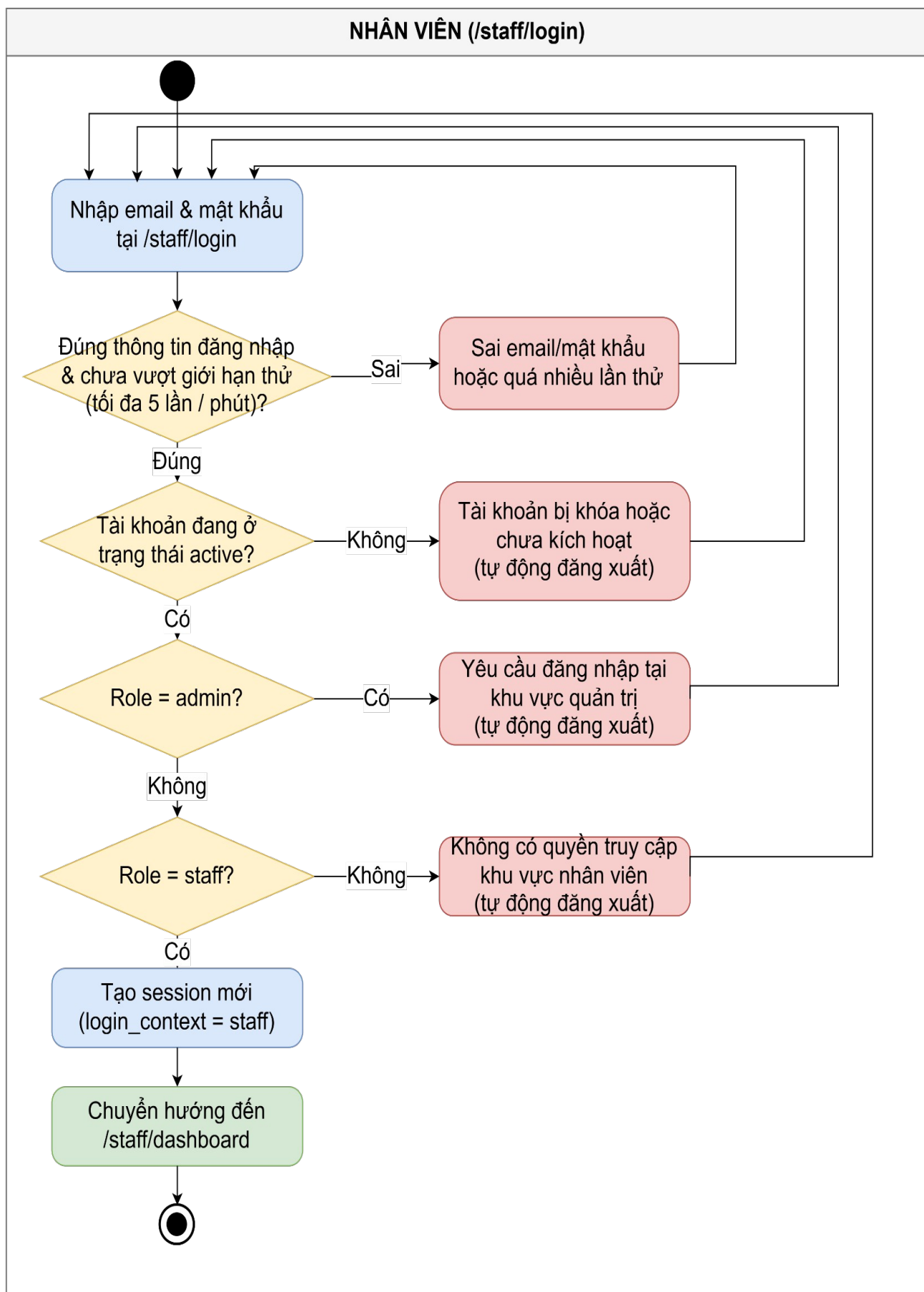
Hình 3.7.2.2: Sơ đồ hoạt động chức năng đăng nhập nhân viên
