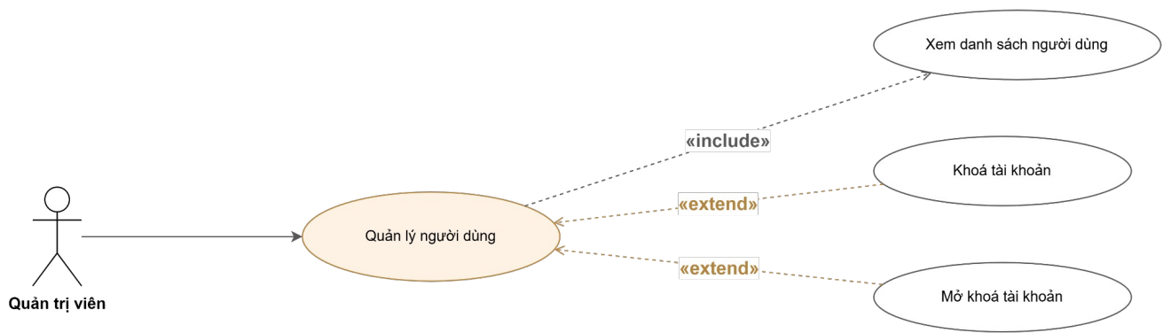
Hình 3.4.2.27: Sơ đồ Use case — Quản lý người dùng
