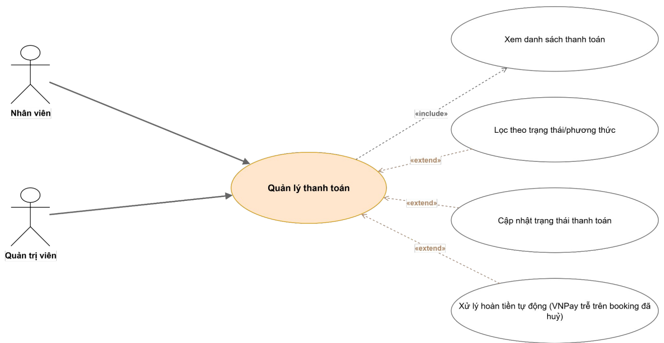
Hình 3.4.2.16: Sơ đồ Use case — Quản lý thanh toán
