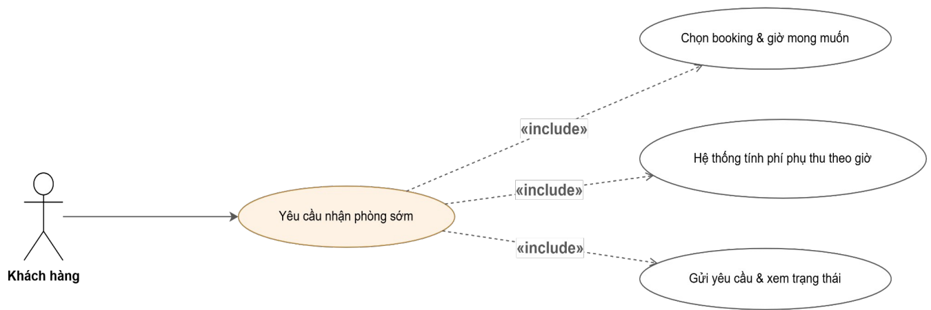
Hình 3.4.2.8: Sơ đồ Use case — Yêu cầu nhận phòng sớm
