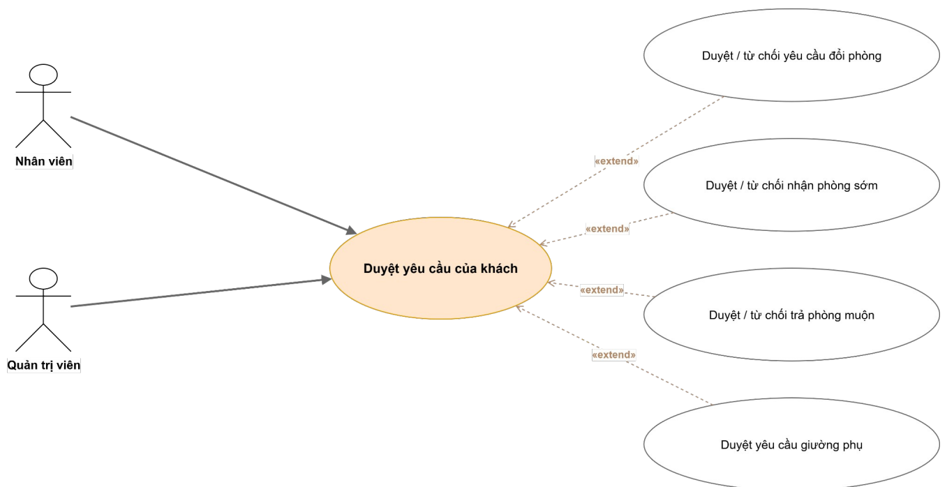
Hình 3.4.2.17: Sơ đồ Use case — Duyệt yêu cầu phát sinh
