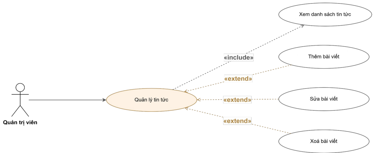
Hình 3.4.2.30: Sơ đồ Use case — Quản lý tin tức
