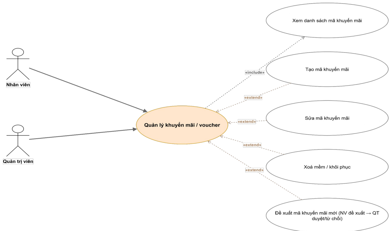
Hình 3.4.2.23: Sơ đồ Use case — Quản lý khuyến mãi
