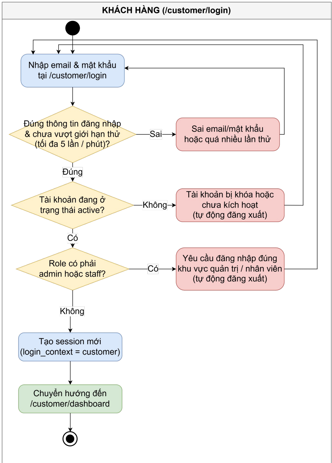
Hình 3.7.2.1: Sơ đồ hoạt động chức năng đăng nhập khách hàng
