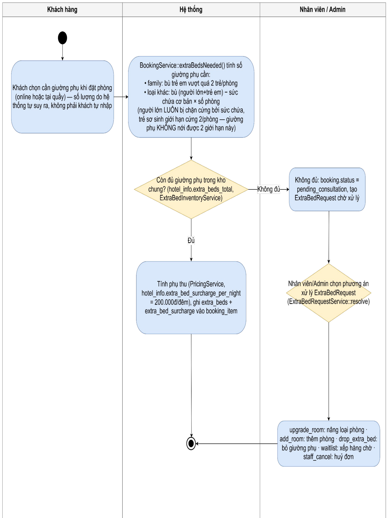
Hình 3.7.21: Sơ đồ hoạt động chức năng đặt giường phụ
