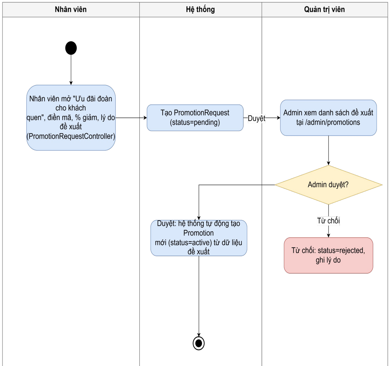
Hình 3.7.24: Sơ đồ hoạt động chức năng yêu đề xuất & duyệt mã khuyến mãi mới
