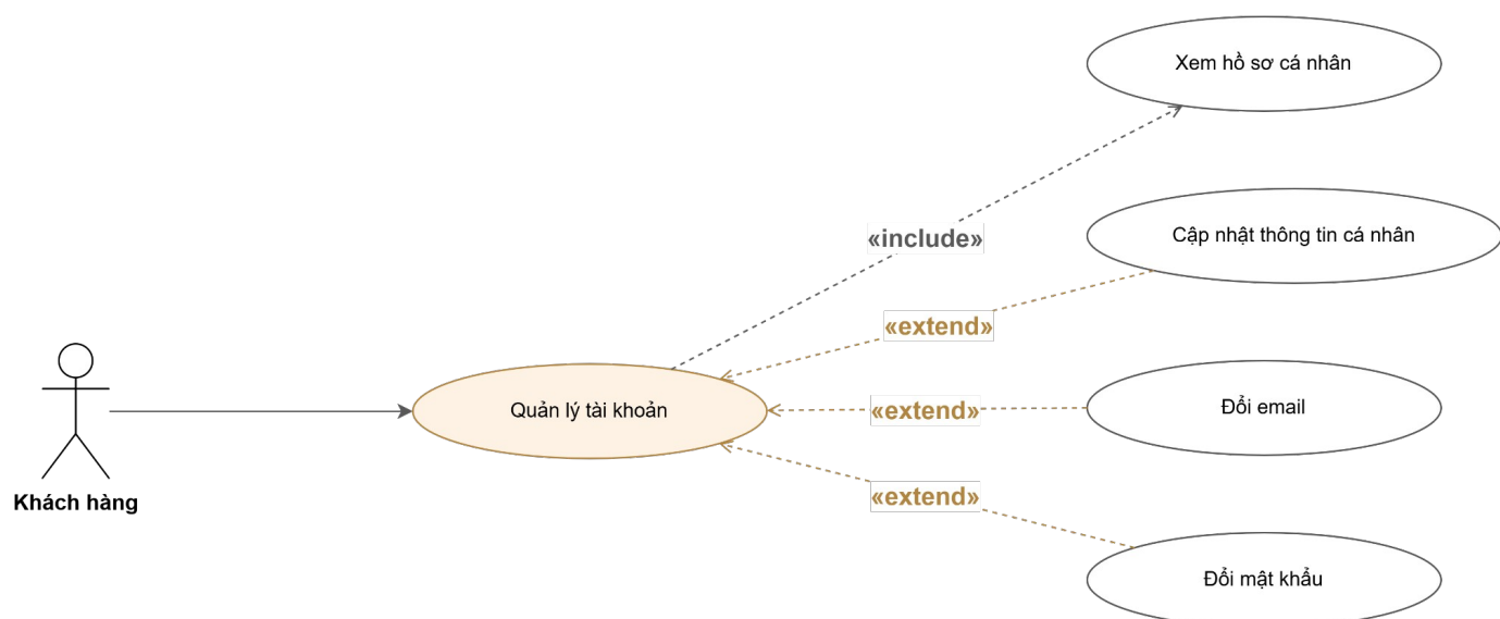
Hình 3.4.2.4: Sơ đồ Use case — Quản lý tài khoản cá nhân
