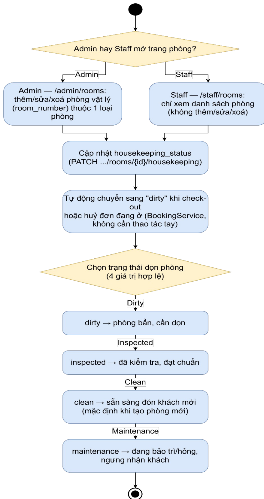
Hình 3.7.11: Sơ đồ hoạt động chức năng quản lý phòng vật lý & housekeeping
