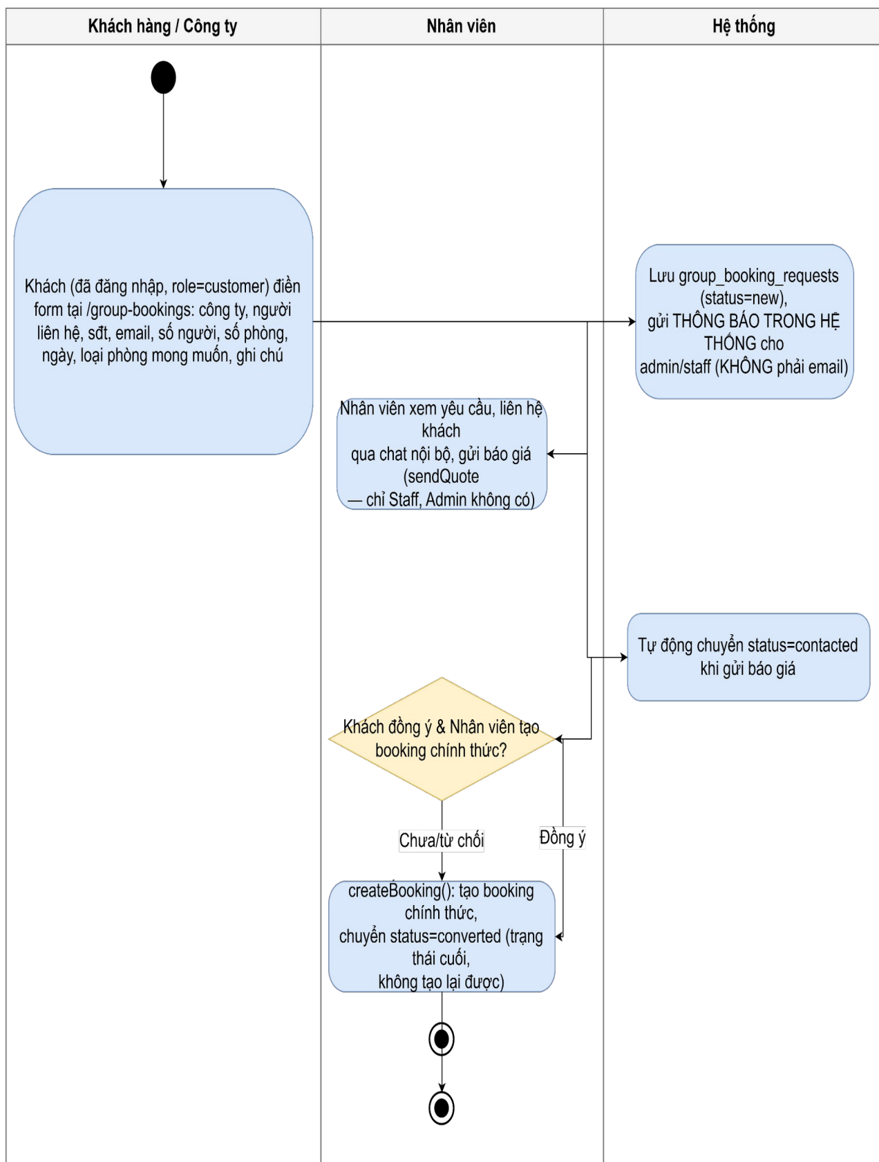
Hình 3.7.19 – Sơ đồ hoạt động chức năng yêu cầu đặt đoàn / nhóm
