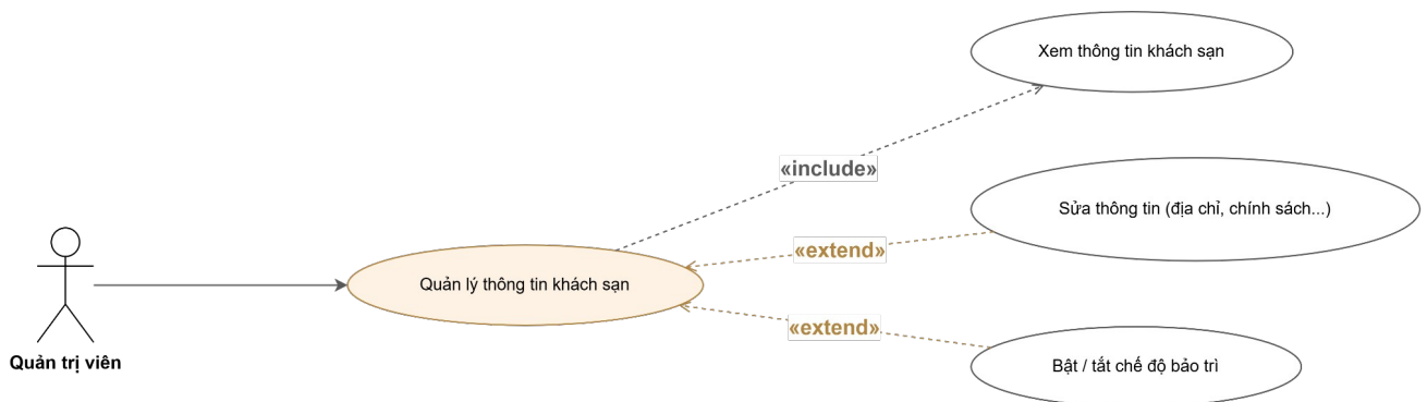
Hình 3.4.2.26: Sơ đồ Use case — Quản lý thông tin khách sạn
