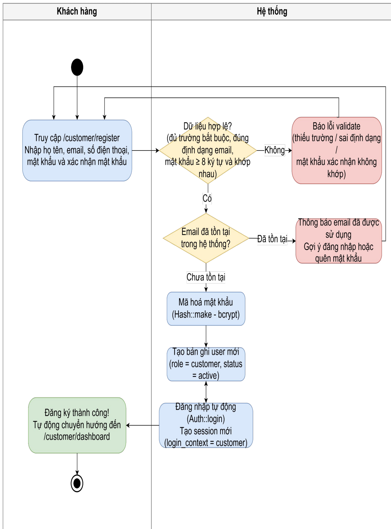
Hình 3.7.1: Sơ đồ hoạt động chức năng đăng ký tài khoản
