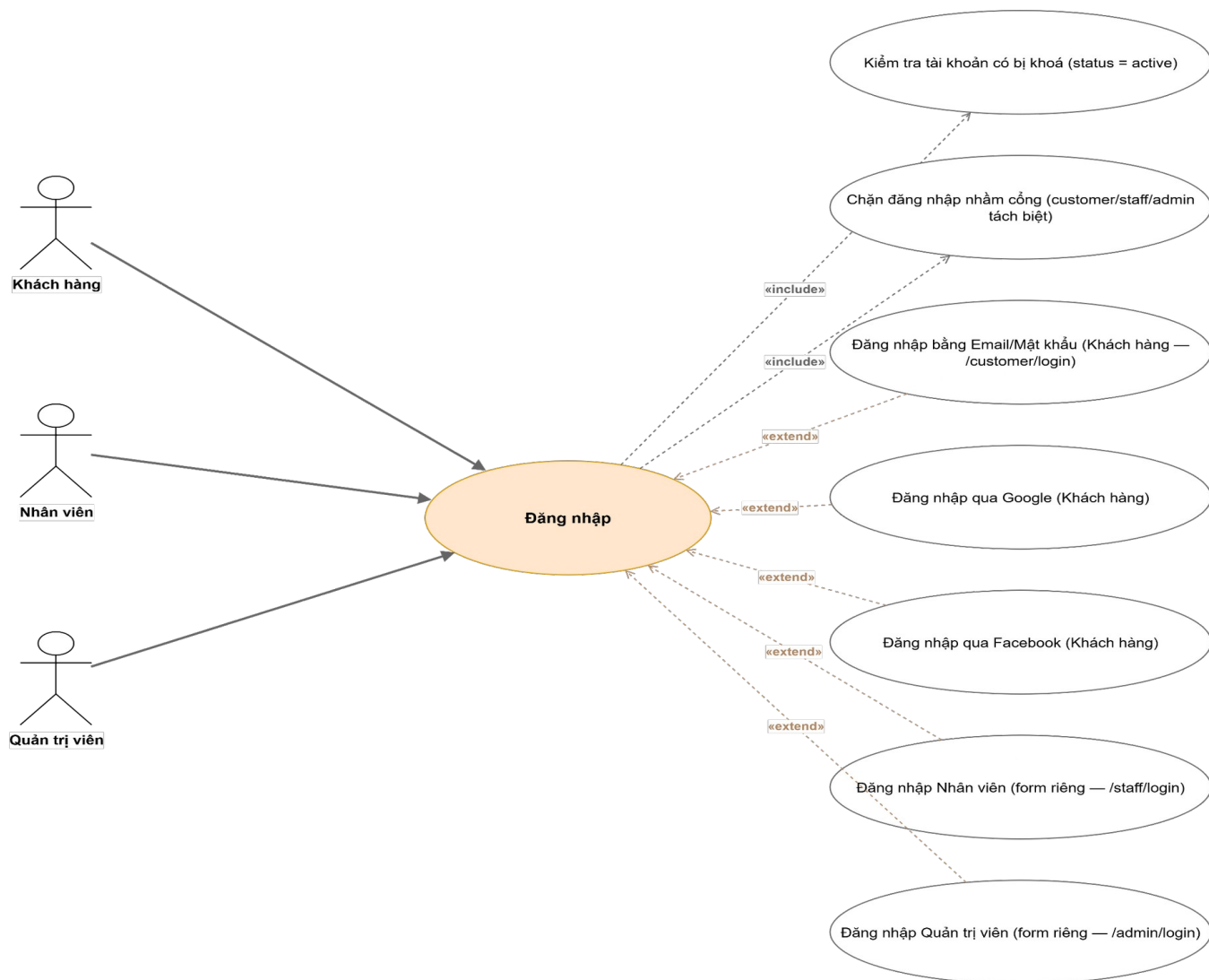
Hình 3.4.2.1: Sơ đồ Use case — Đăng nhập
