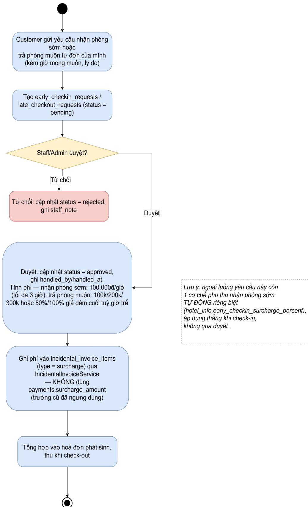
Hình 3.7.20: Sơ đồ hoạt động chức năng yêu cầu nhận phòng sớm / trả phòng muộn
