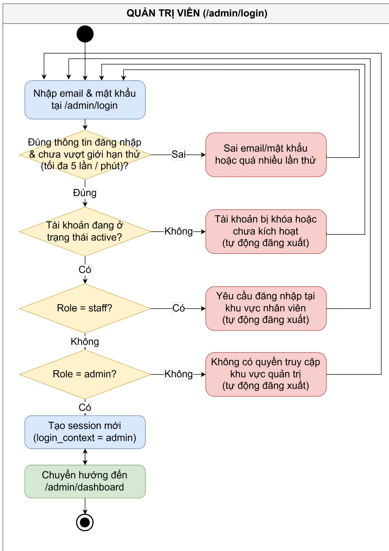
Hình 3.7.2.3: Sơ đồ hoạt động chức năng đăng nhập admin
