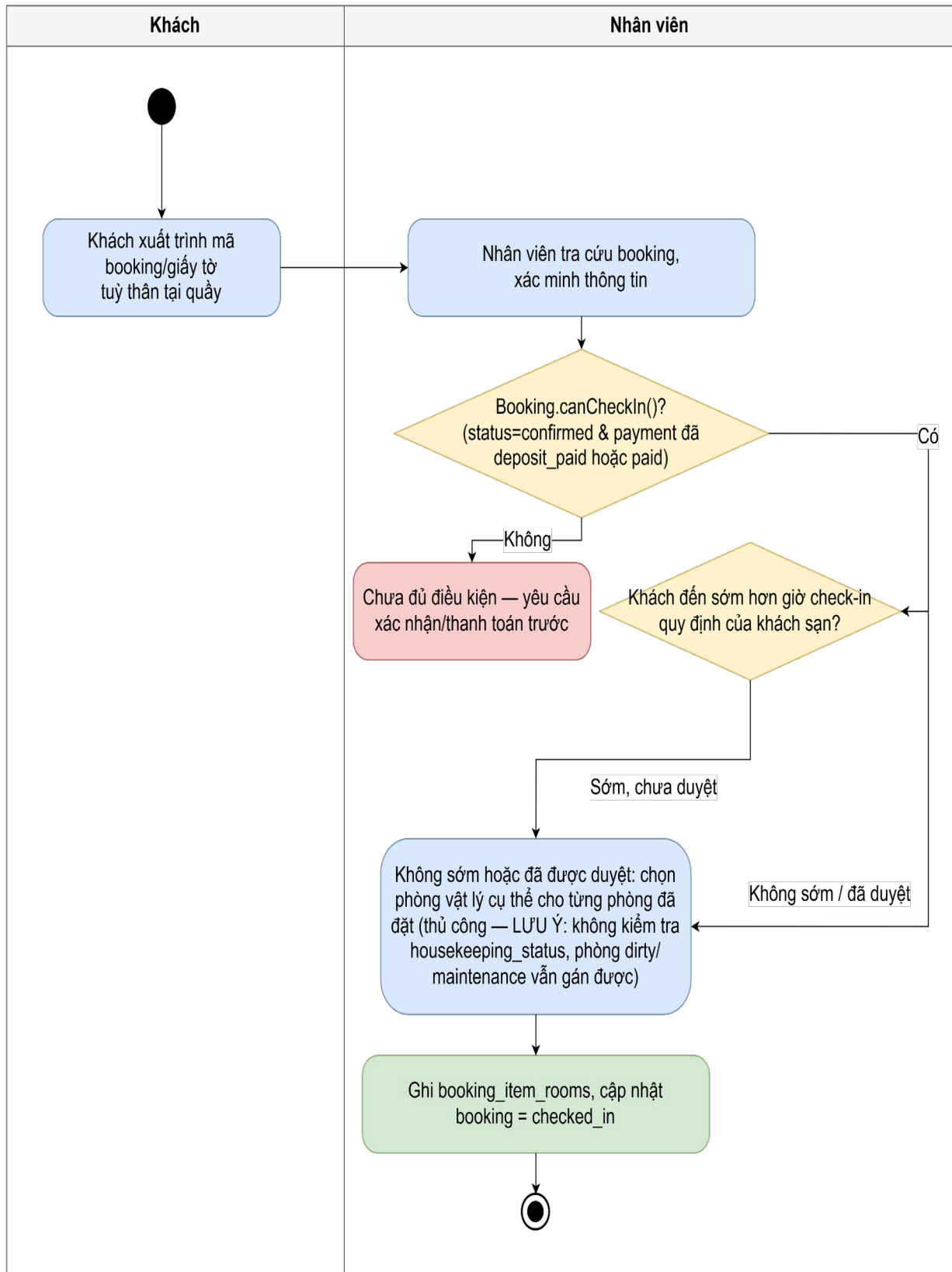
Hình 3.7.16: Sơ đồ hoạt động chức năng check-in
