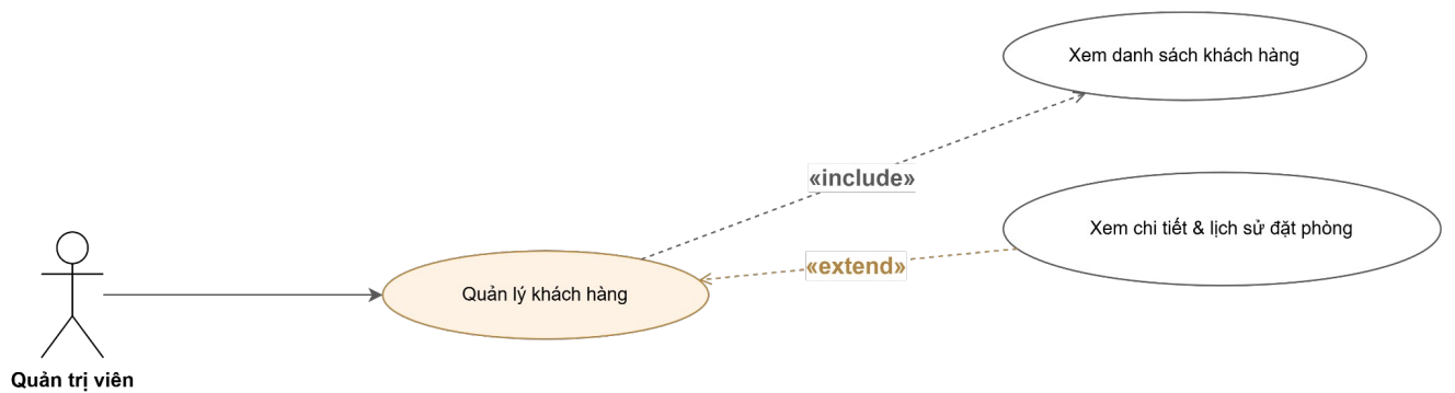
Hình 3.4.2.28: Sơ đồ Use case — Quản lý khách hàng
