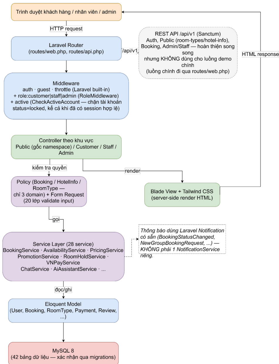
Hình 4.1 – Sơ đồ kiến trúc hệ thống Homi
