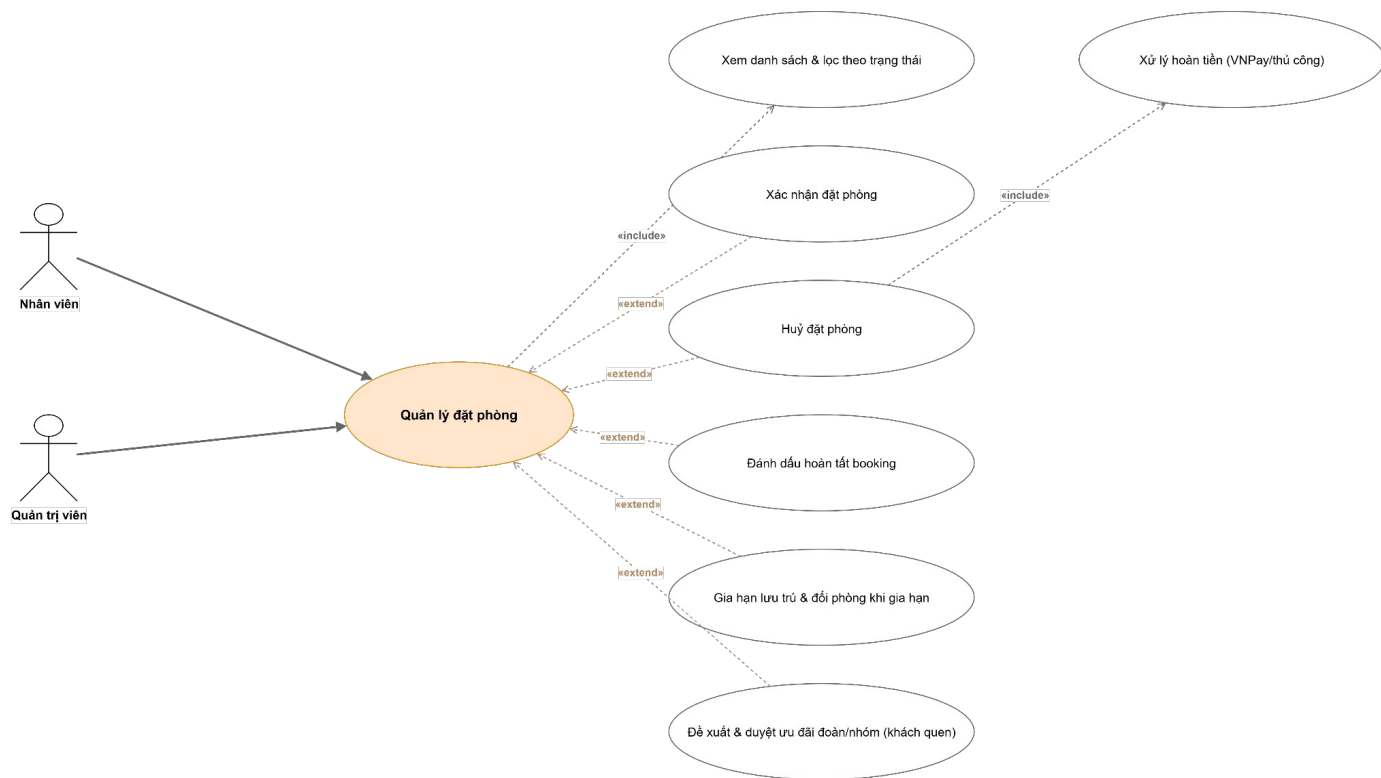
Hình 3.4.2.14: Sơ đồ Use case — Quản lý đặt phòng
