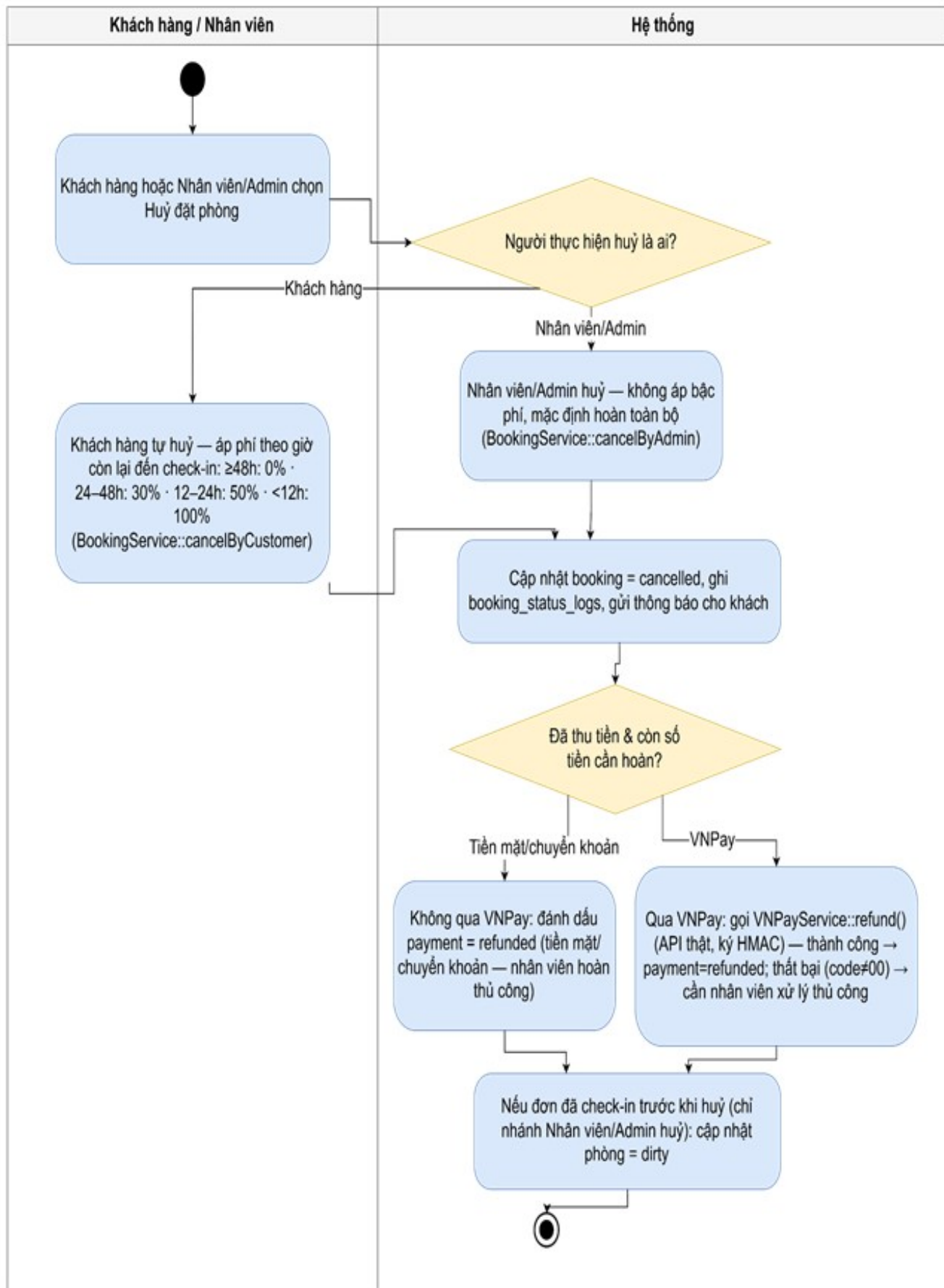
Hình 3.7.5: Sơ đồ hoạt động chức năng hủy booking và hoàn tiền
