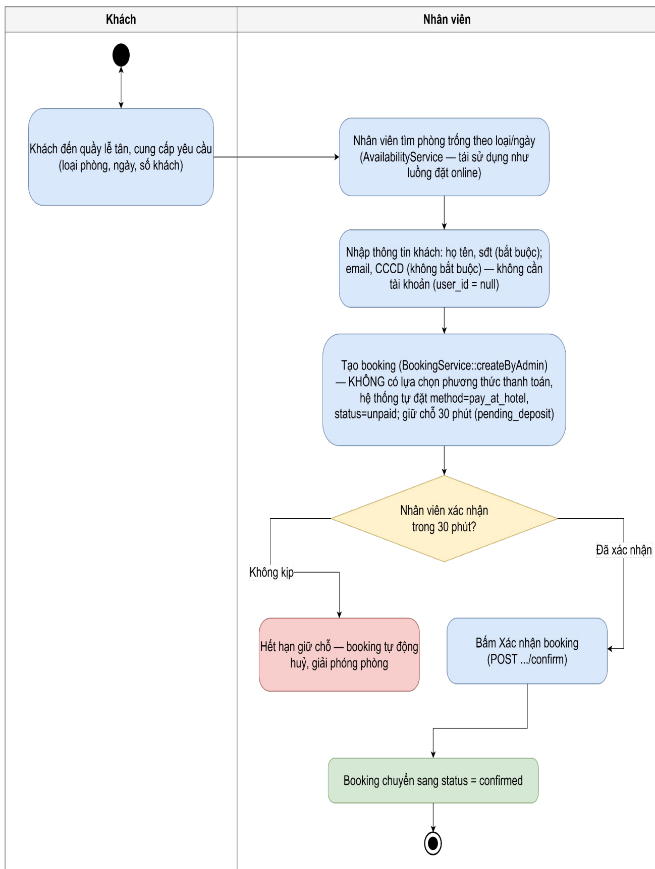
Hình 3.7.4: Sơ đồ hoạt động chức năng đặt phòng tại quầy (staff, walk-in)
