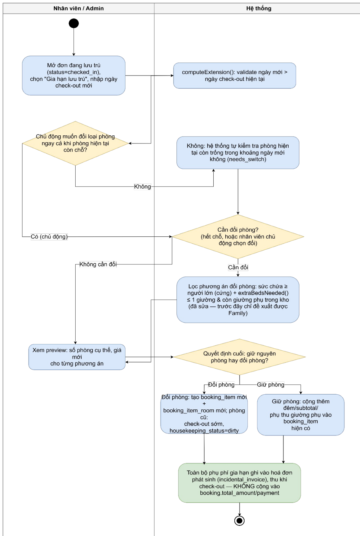
Hình 3.7.22: Sơ đồ hoạt động chức năng gia hạn lưu trú / đổi phòng khi gia hạn
