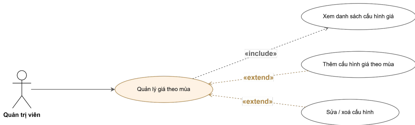
Hình 3.4.2.24: Sơ đồ Use case — Quản lý giá theo mùa
