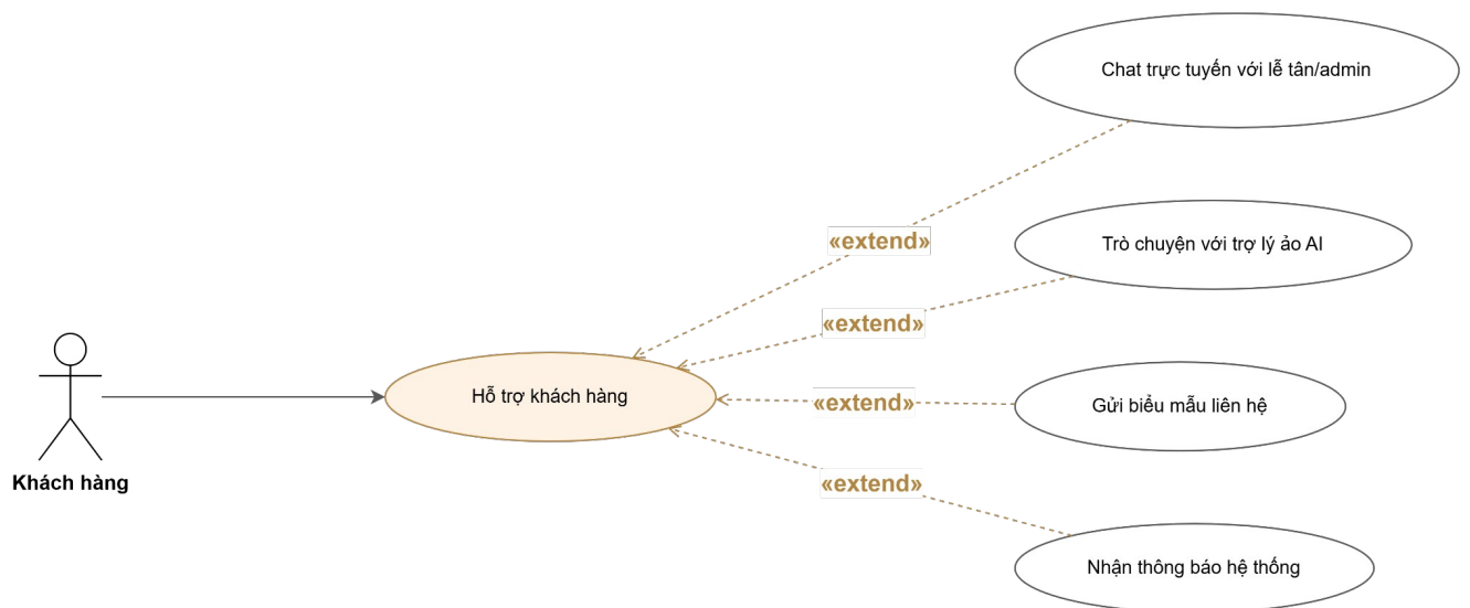
Hình 3.4.2.11: Sơ đồ Use case — Hỗ trợ & Liên hệ
