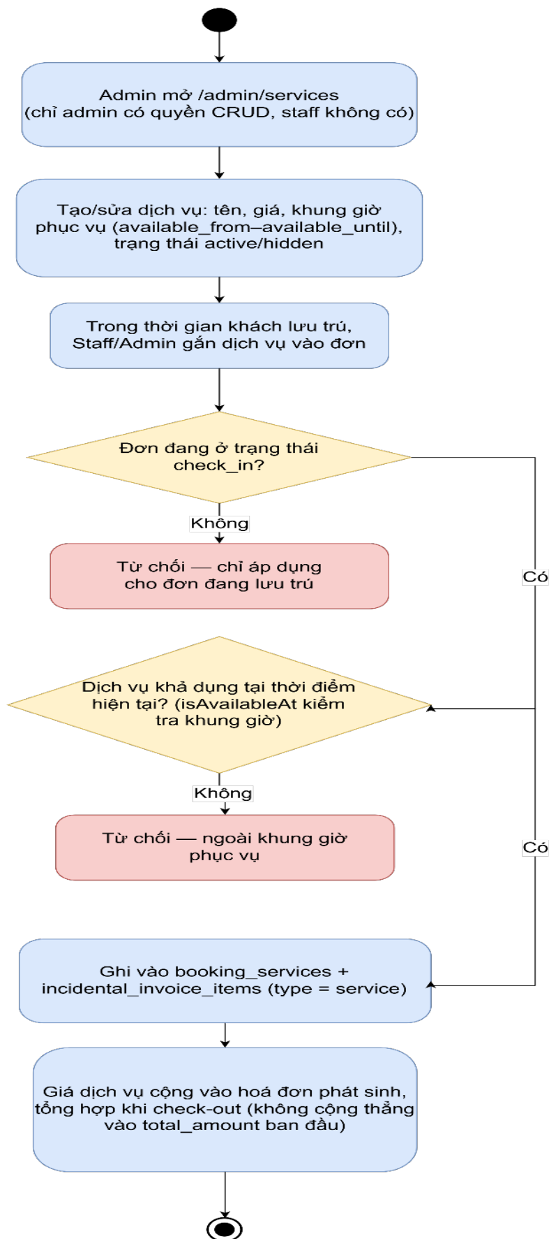
Hình 3.7.13: Sơ đồ hoạt động chức năng quản lý dịch vụ phát sinh
