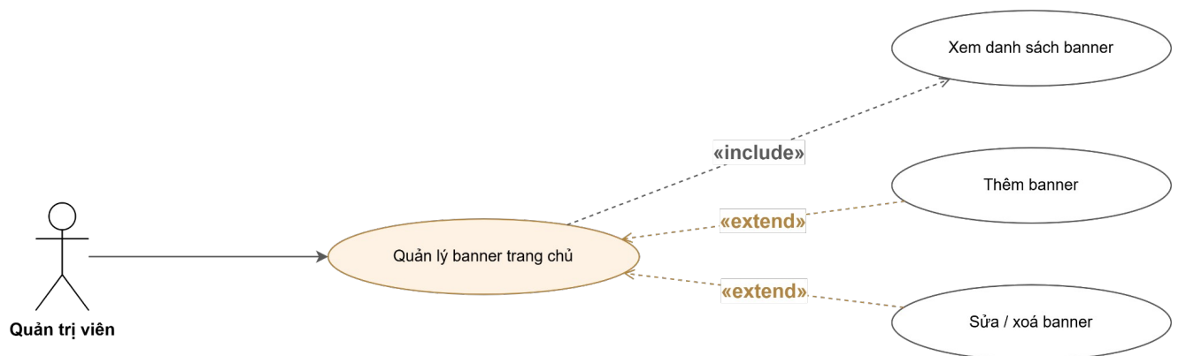
Hình 3.4.2.25: Sơ đồ Use case — Quản lý banner
