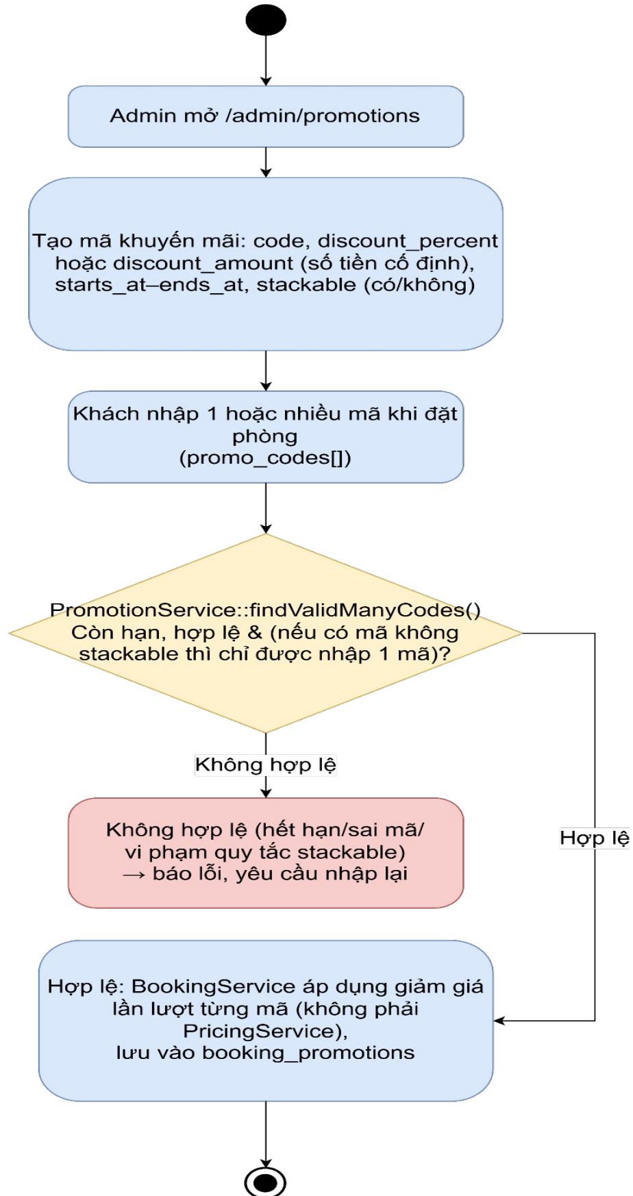
Hình 3.7.14: Sơ đồ hoạt động chức năng quản lý khuyến mãi
