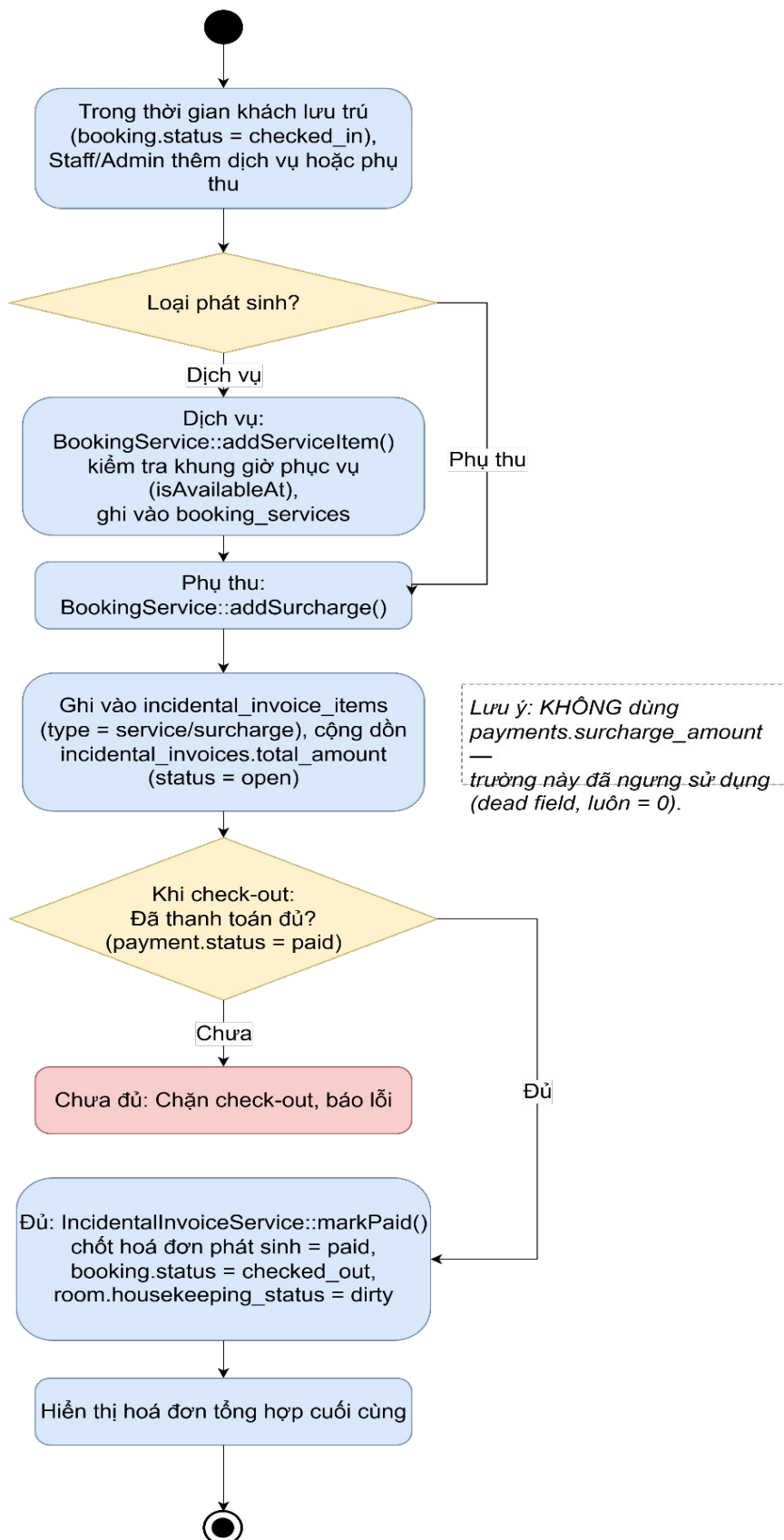
Hình 3.7.8 – Sơ đồ hoạt động chức năng quản lý hoá đơn phát sinh nội bộ
