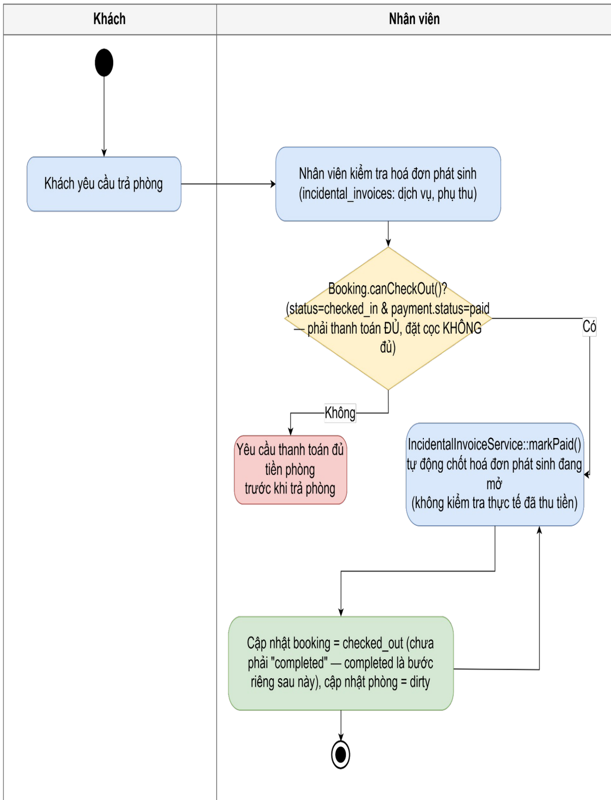
Hình 3.7.17 : Sơ đồ hoạt động chức năng check-out
