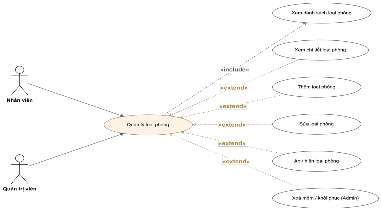
Hình 3.4.2.20: Sơ đồ Use case — Quản lý loại phòng
