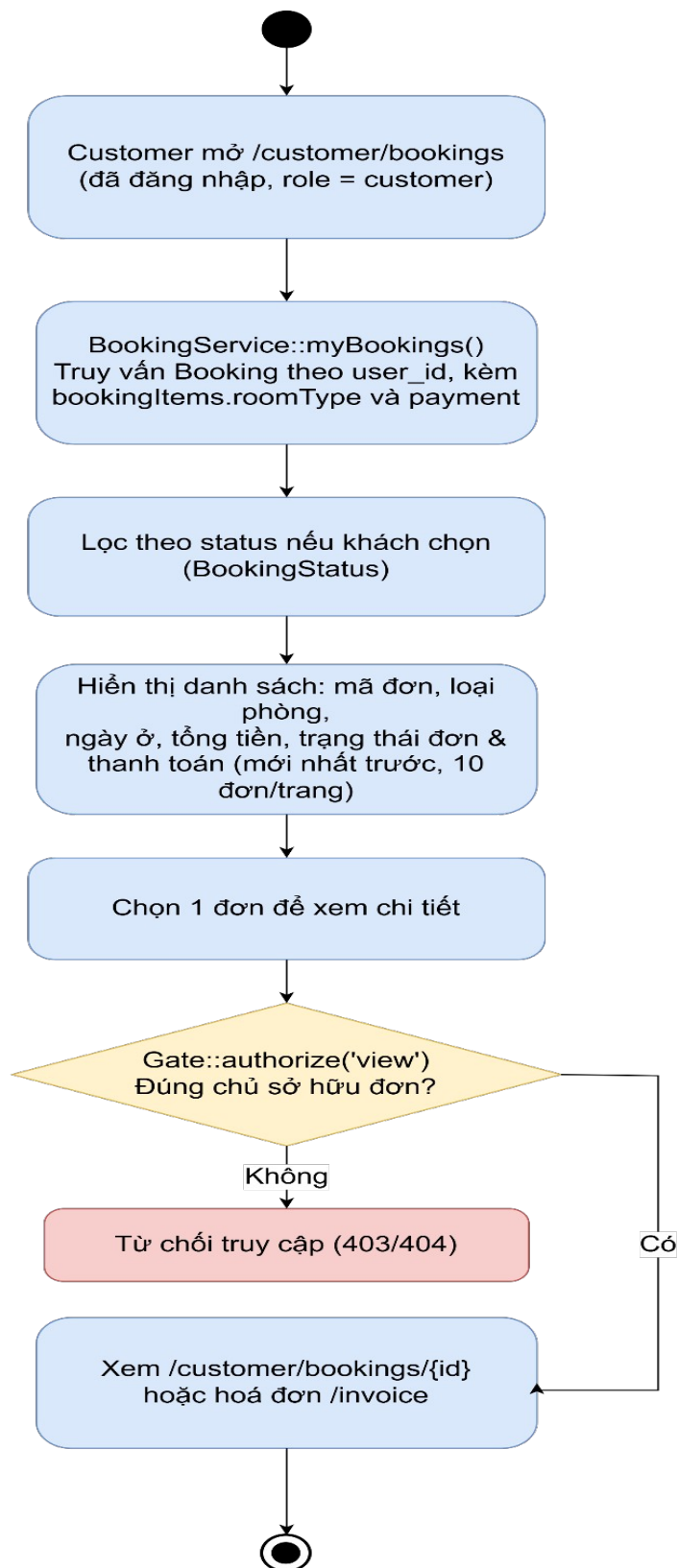
Hình 3.7.6 – Sơ đồ hoạt động chức năng xem lịch sử đặt phòng (khách hàng)
