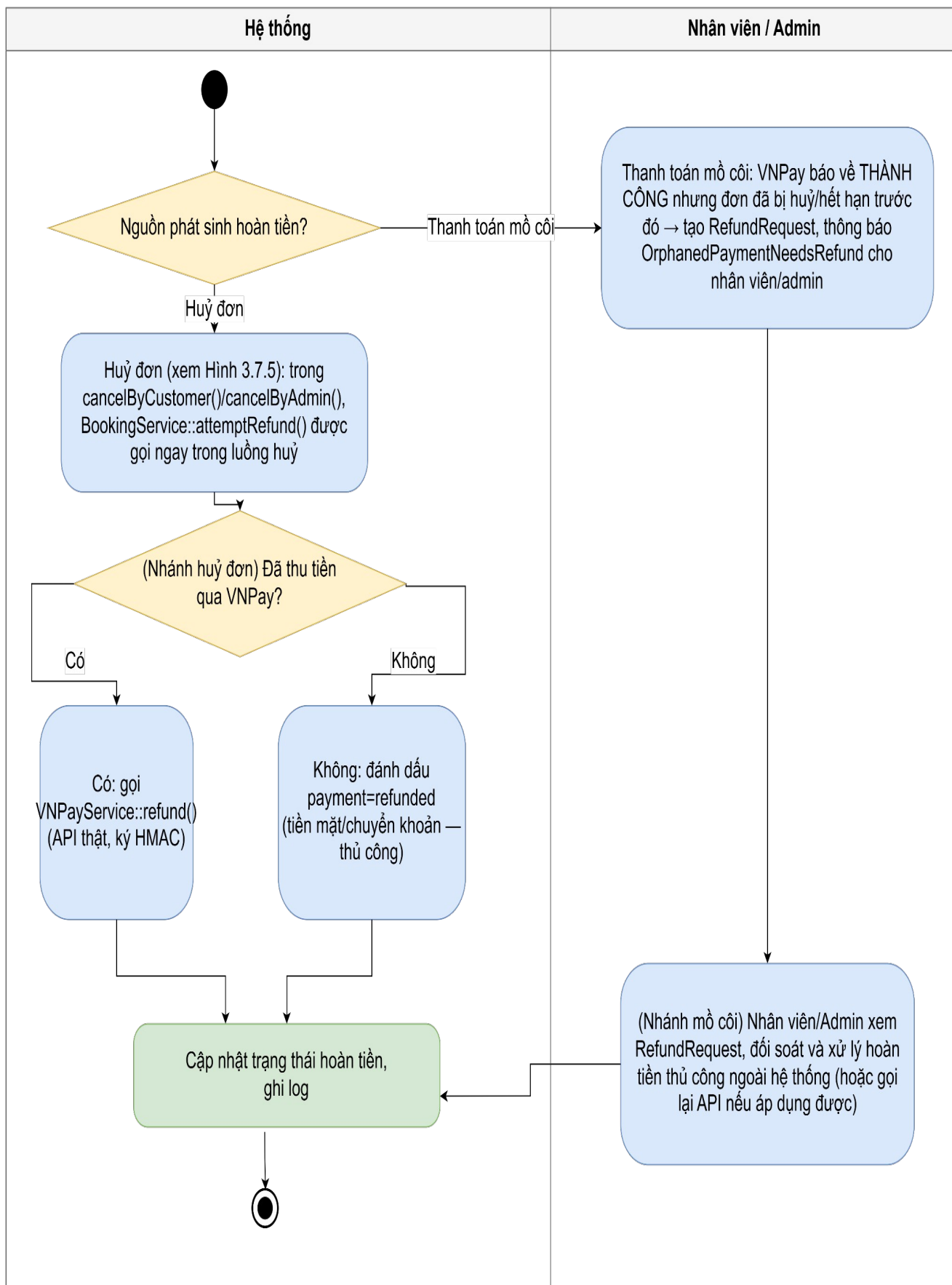
Hình 3.7.23: Sơ đồ hoạt động chức năng xử lý hoàn tiền
