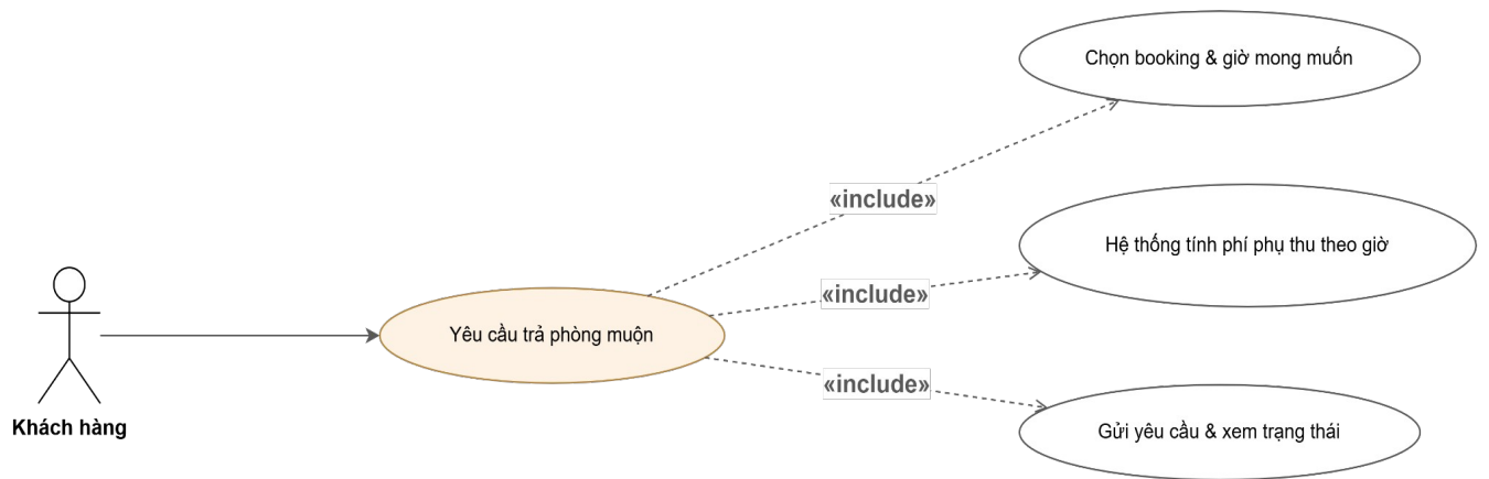
Hình 3.4.2.9: Sơ đồ Use case — Yêu cầu trả phòng muộn
