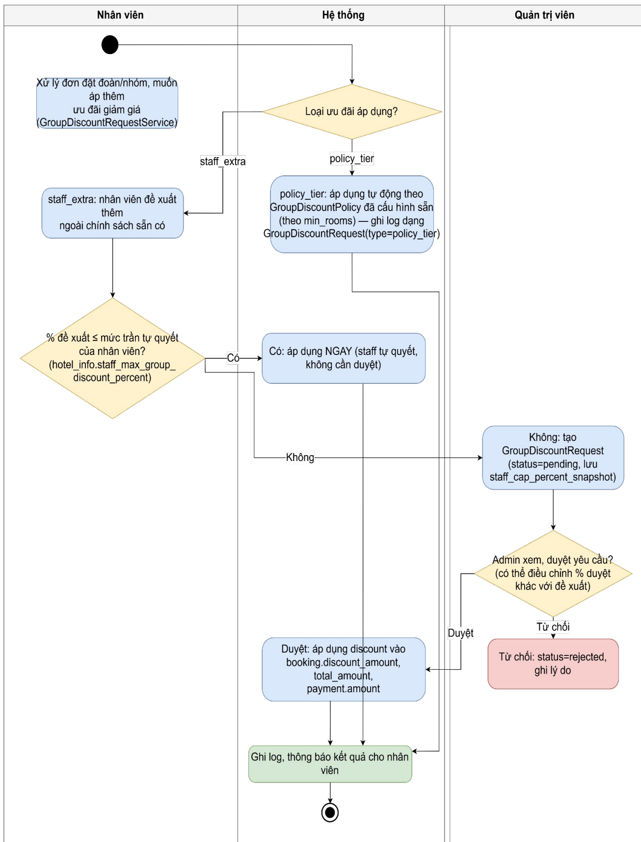
Hình 3.7.25: Sơ đồ hoạt động chức năng yêu đề xuất & duyệt ưu đãi đặt đoàn nhóm
