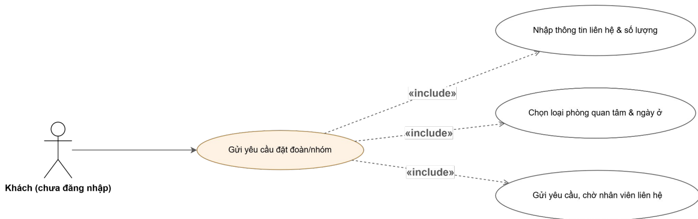
Hình 3.4.2.12: Sơ đồ Use case — Đặt đoàn / nhóm
