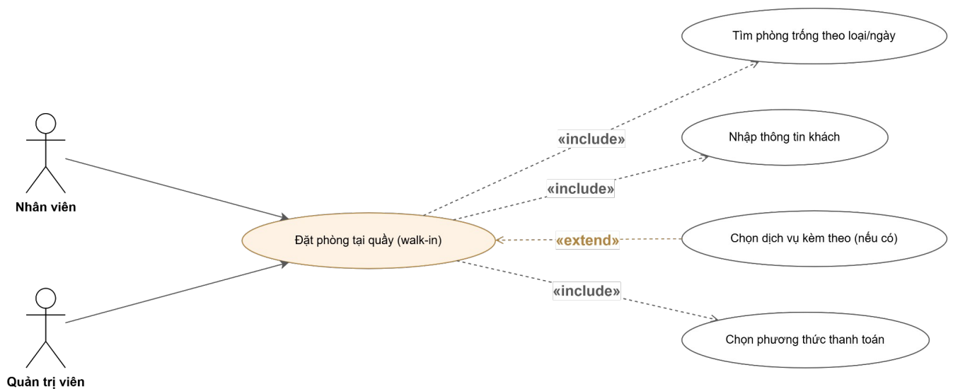
Hình 3.4.2.13: Sơ đồ Use case — Đặt phòng tại quầy
