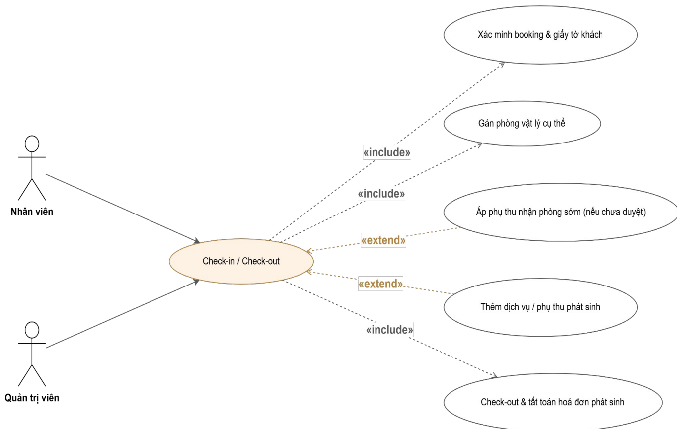
Hình 3.4.2.15: Sơ đồ Use case — Check-in / Check-out
