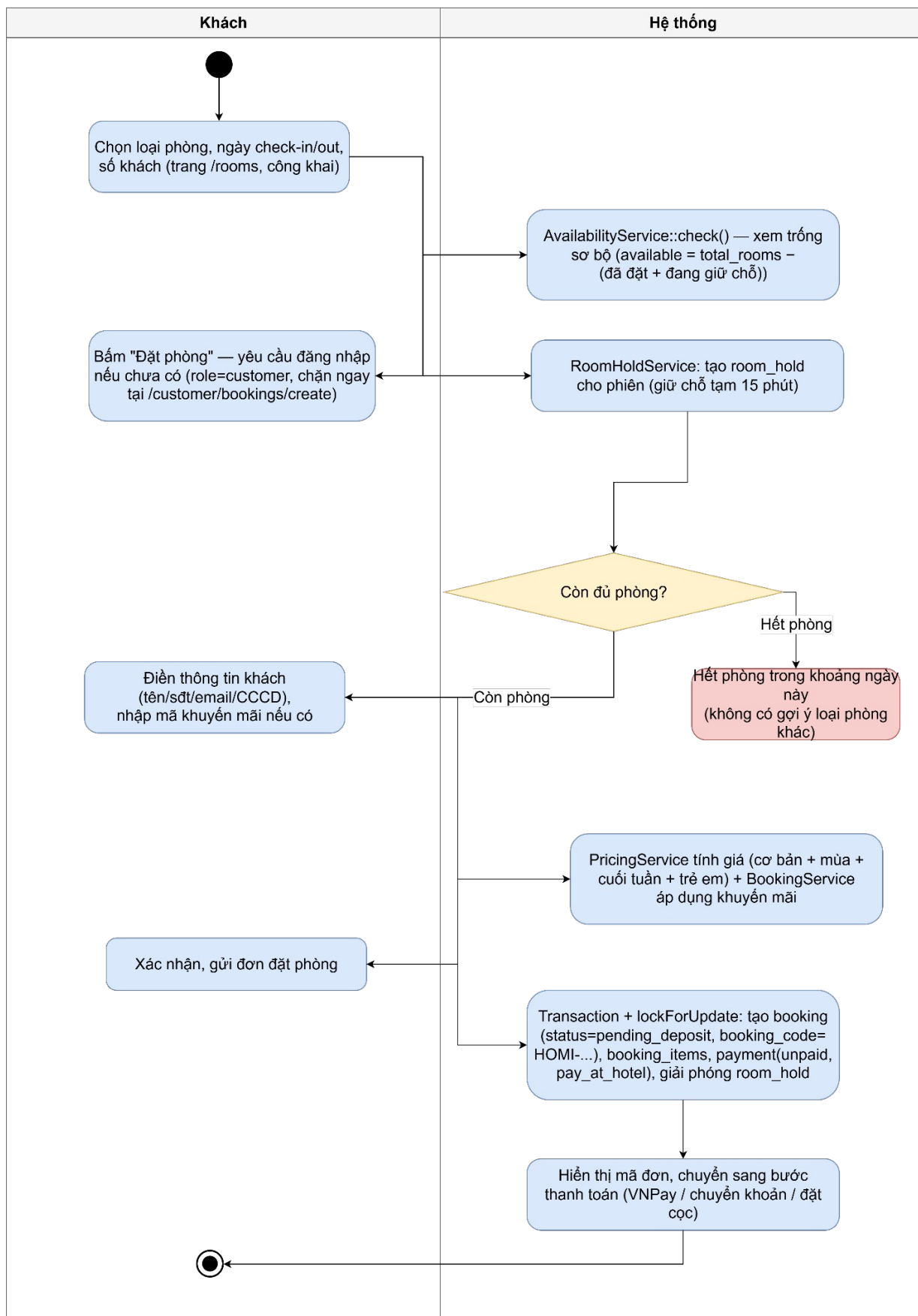
Hình 3.7.3: Sơ đồ hoạt động chức năng đặt phòng online (khách hàng)
