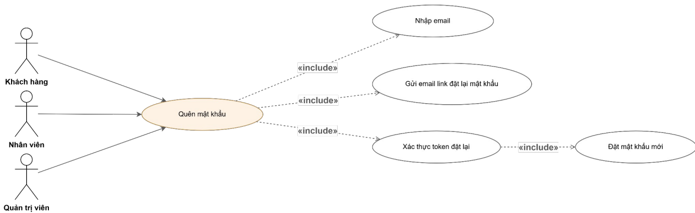
Hình 3.4.2.3: Sơ đồ Use case — Quên mật khẩu
