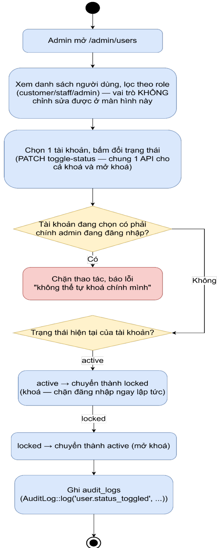
Hình 3.7.12: Sơ đồ hoạt động chức năng quản lý người dùng & phân quyền
