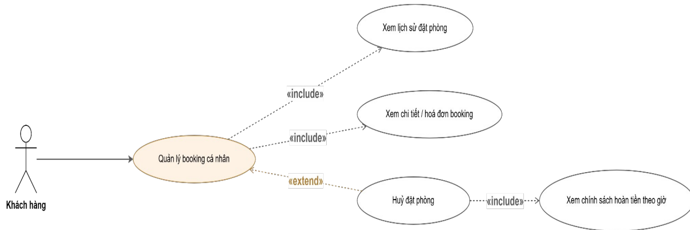
Hình 3.4.2.6: Sơ đồ Use case — Quản lý đặt phòng của tôi
