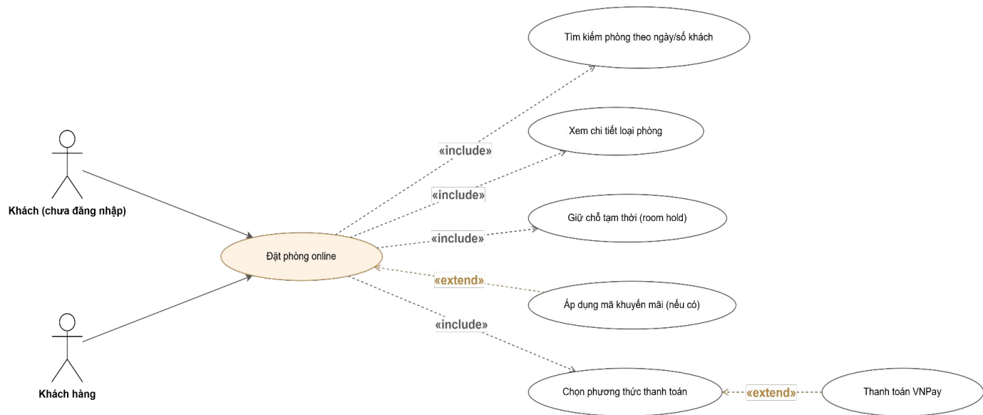
Hình 3.4.2.5: Sơ đồ Use case — Đặt phòng online
