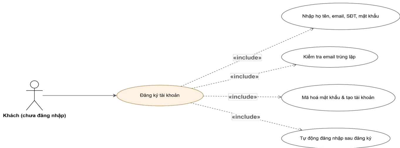
Hình 3.4.2.2: Sơ đồ Use case — Đăng ký
