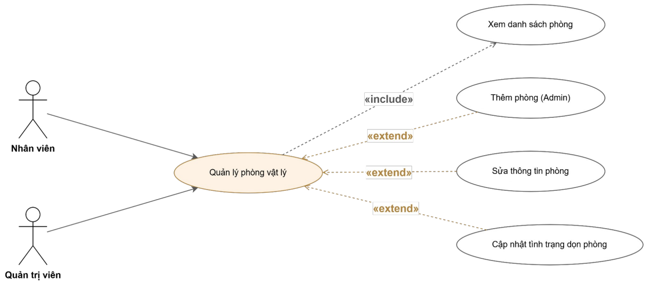
Hình 3.4.2.21: Sơ đồ Use case — Quản lý phòng
