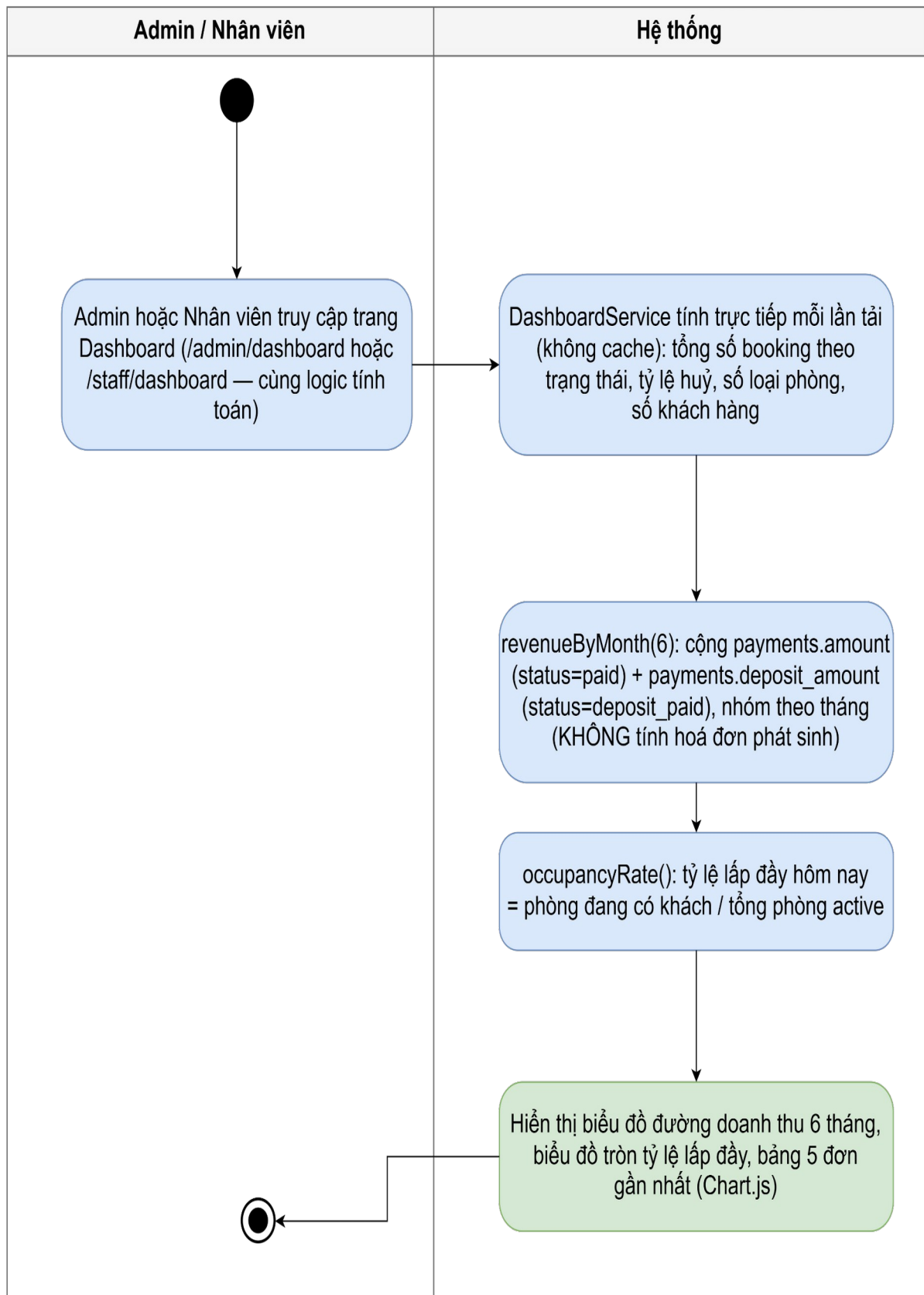
Hình 3.7.15: Sơ đồ hoạt động chức năng dashboard thống kê doanh thu
