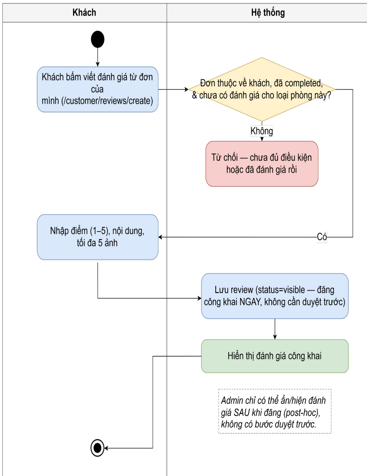
Hình 3.7.18: Sơ đồ hoạt động chức năng viết đánh giá
