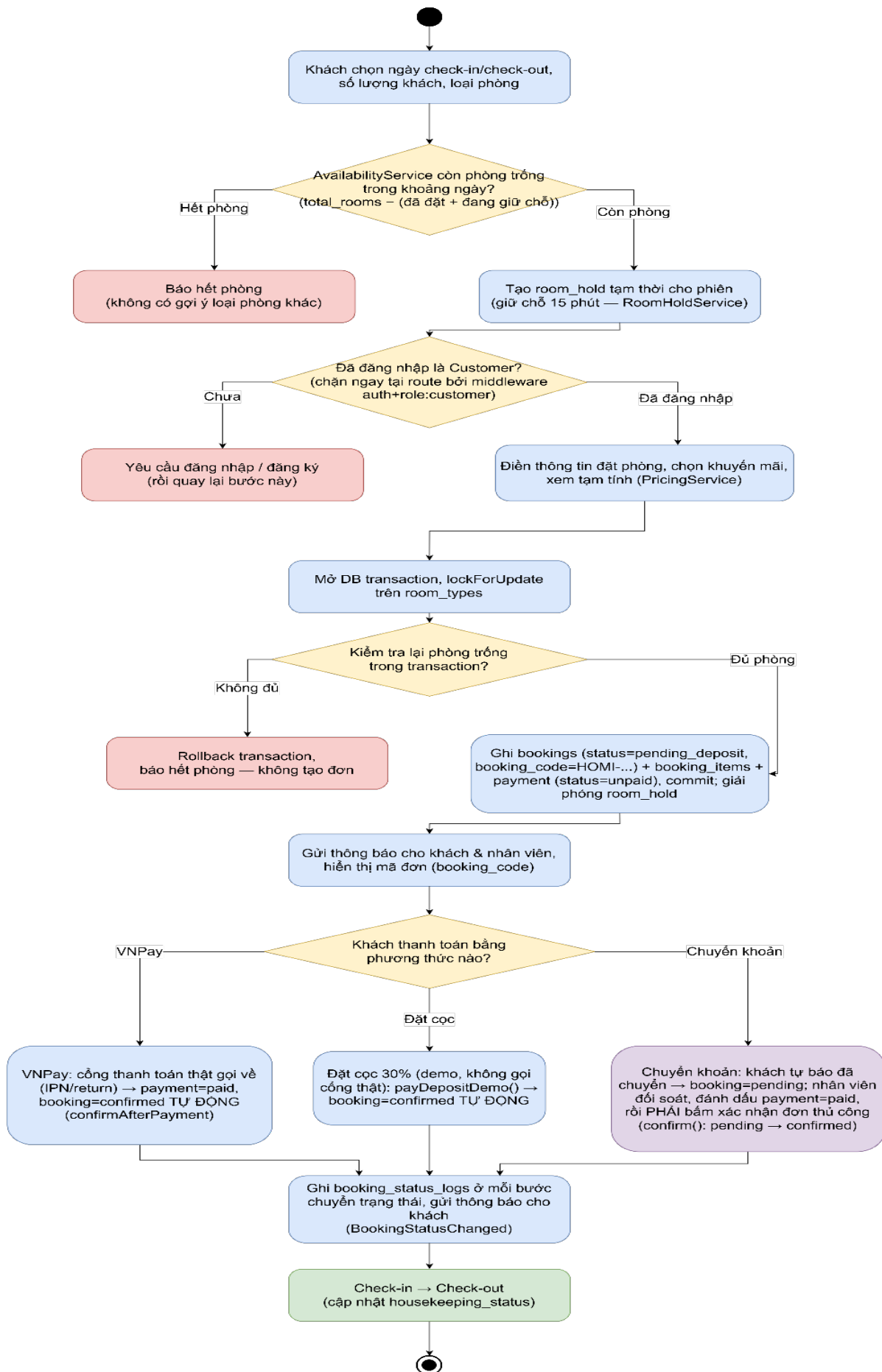
Hình 3.7.0: Sơ đồ hoạt động tổng quan luồng đặt phòng
