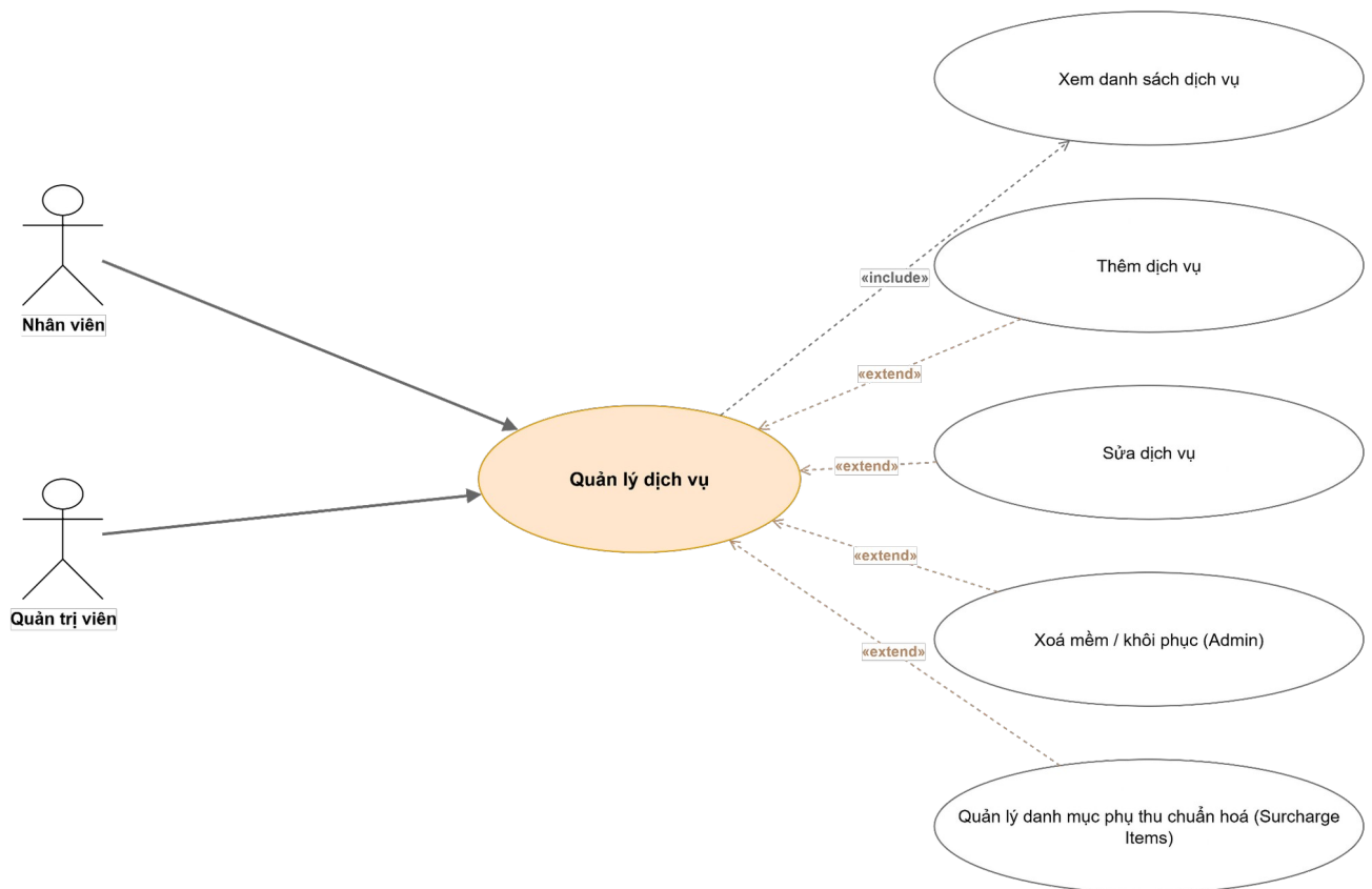
Hình 3.4.2.22: Sơ đồ Use case — Quản lý dịch vụ
