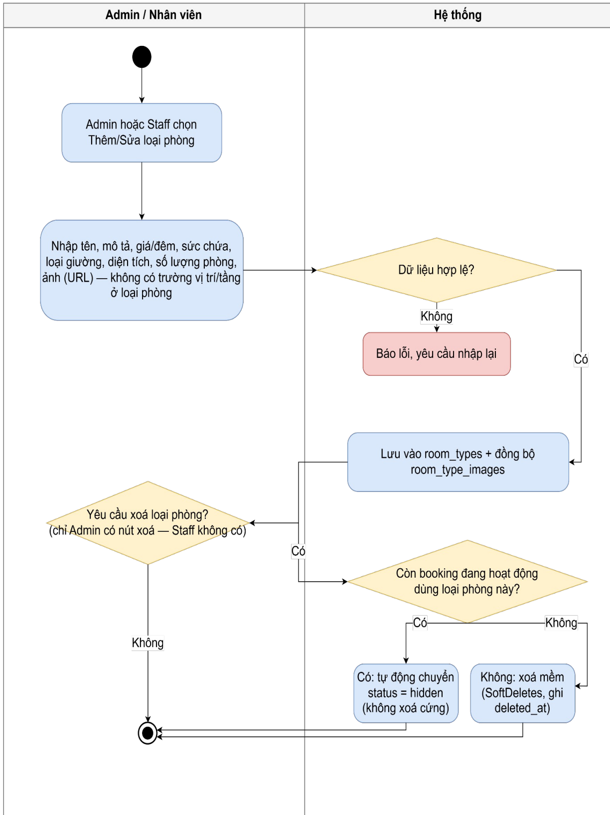
Hình 3.7.10: Sơ đồ hoạt động chức năng quản lý loại phòng (admin/staff)
