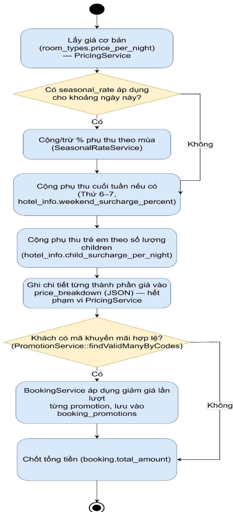
Hình 3.7.7 – Sơ đồ hoạt động chức năng tính toán hoá đơn (PricingService)
