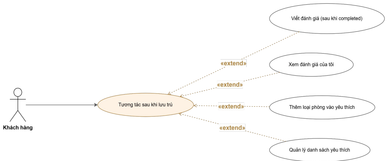
Hình 3.4.2.10: Sơ đồ Use case — Đánh giá & Yêu thích
